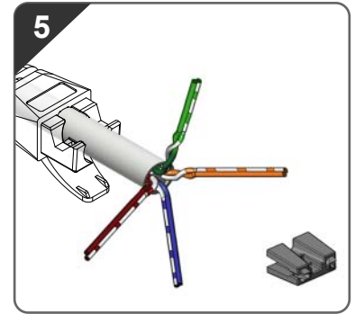
■ Untwist 4 pairs.
