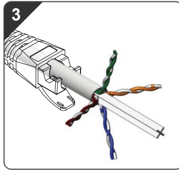
■ Separate 4 pairs.
